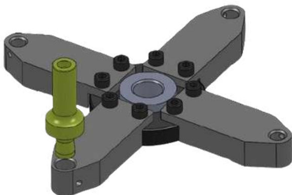
4-ПОЗИЦІЙНА РЕВОЛЬВЕРНА СИСТЕМА З АВТОМАТИЧНИМ ВИЗНАЧЕННЯМ РОБОЧОЇ ПОЗИЦІЇ
